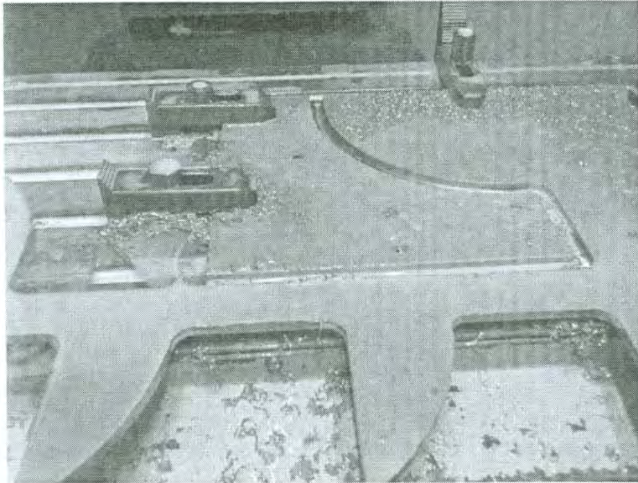
Figura 3.6 Cartagón para Soporte de Estructura.
