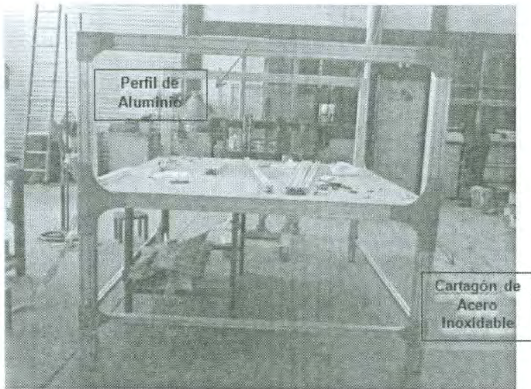
Figura 3.7 Estructura base.
