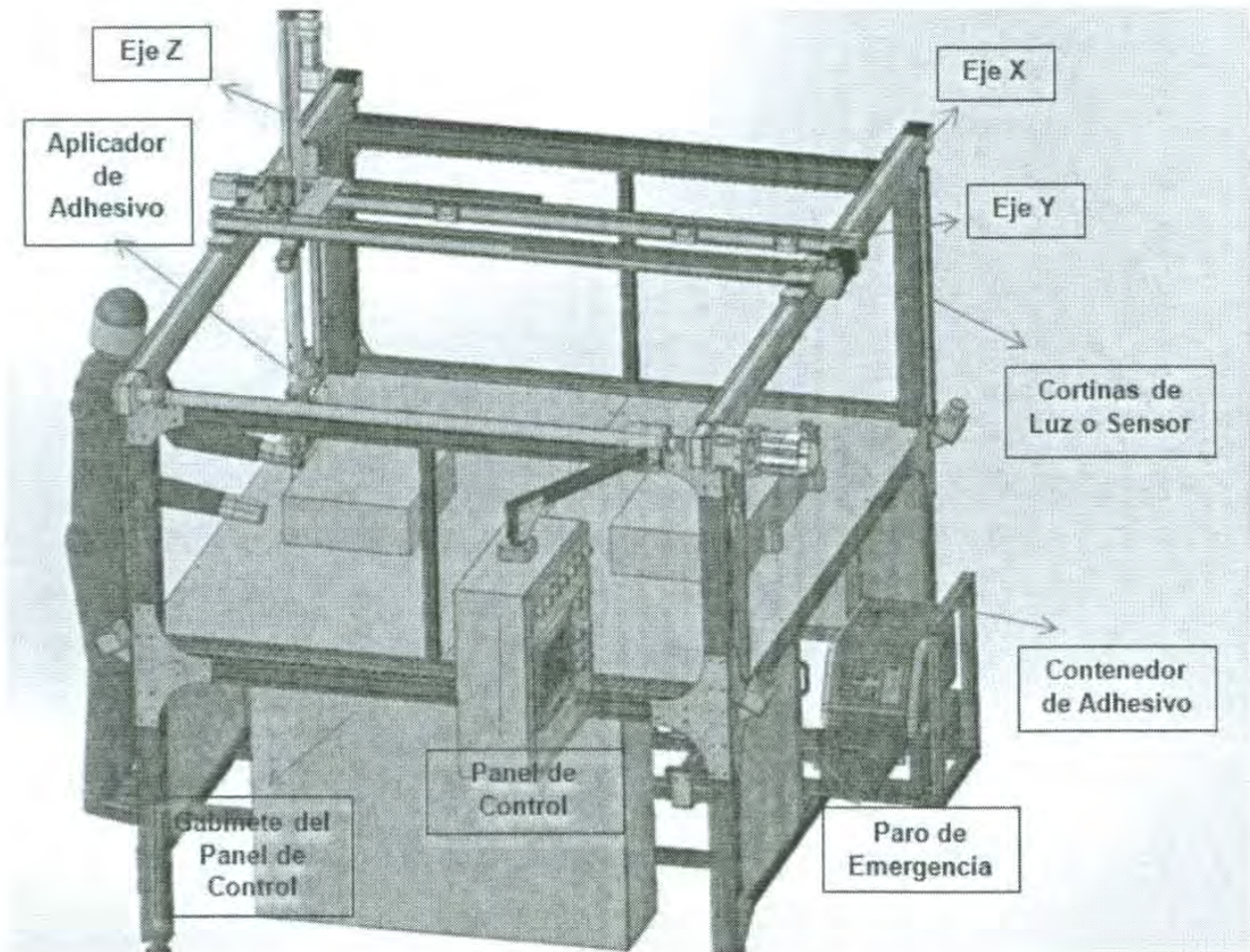
Figura 3.2 Diseño de NG3 XYZ GLUIN SYSTEM.
