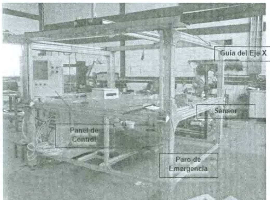
Figura 3.8 Estructura.
