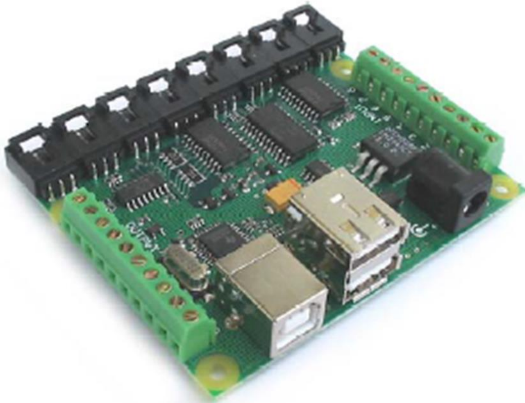
Figura 4.9. Tarjeta de adquisición de datos Phidget Interface Kit 8/8/8. Fuente: Manual Phidget.
