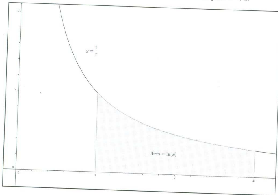
Figura 3.1: Interpretación geométrica de \ln
