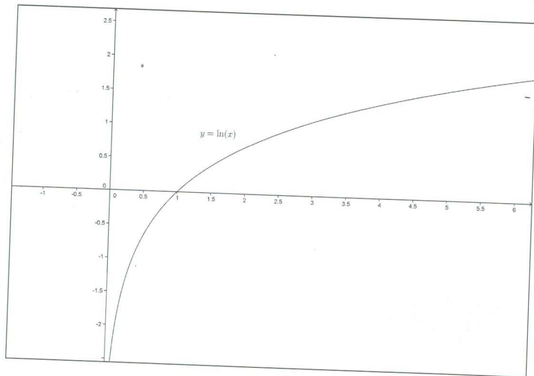
Figura 3.2: Gráfica de la función \ln
