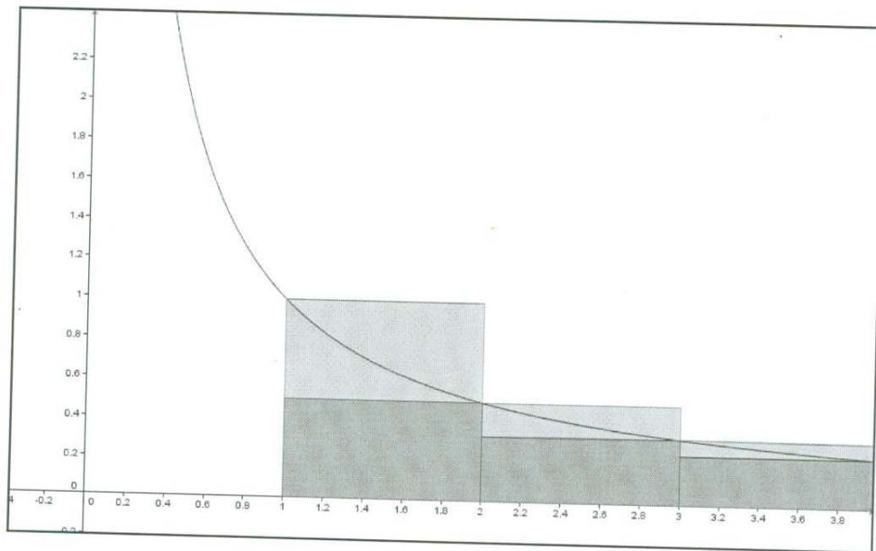
Figura 5.1: Gráfica de la función y = 1/x
